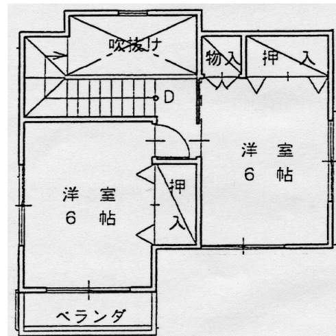
2 階
