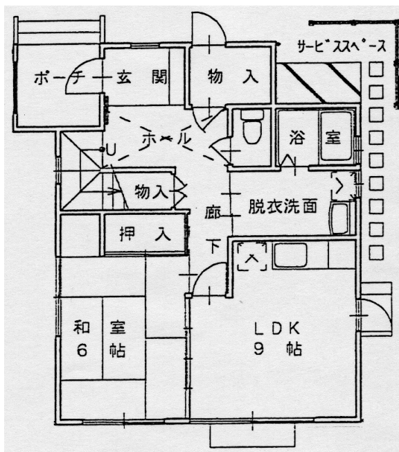
1 階
